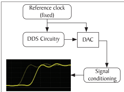
Fig. 1: DDS mode
